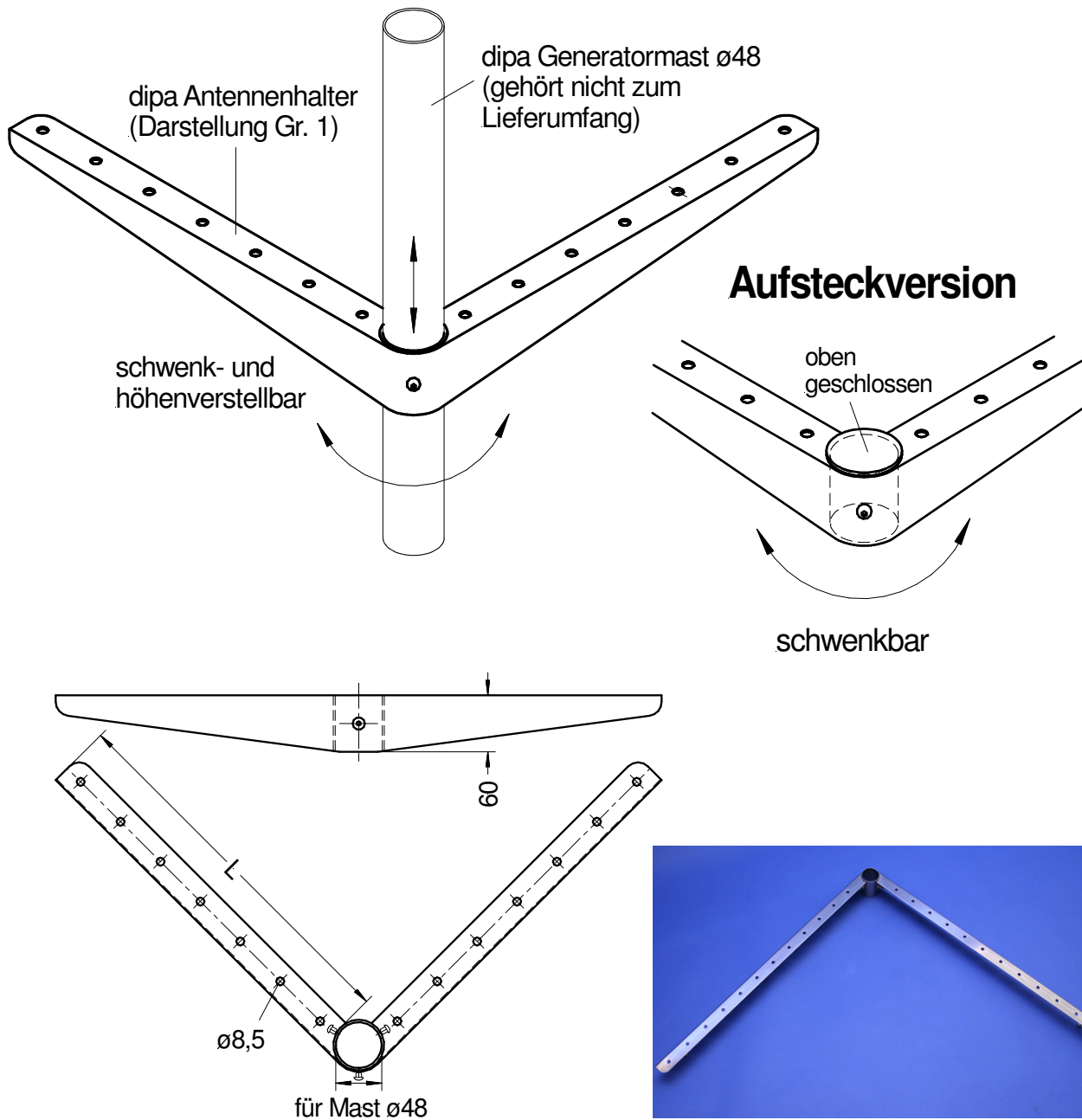
Antennenhalter Gr.2
